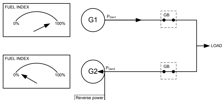
图 2，负频差
