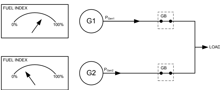
图 1，正频差
